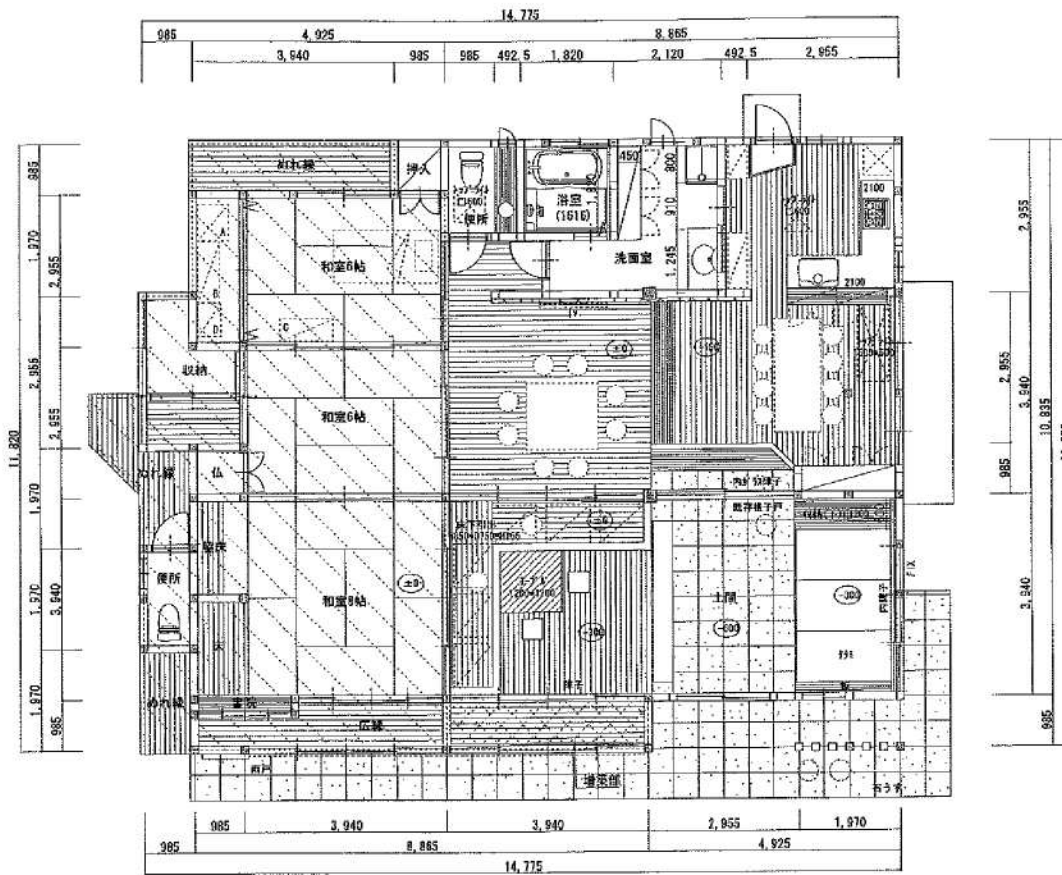
1階平面図 1:100
