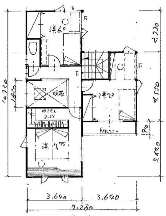
2F. 平面图
